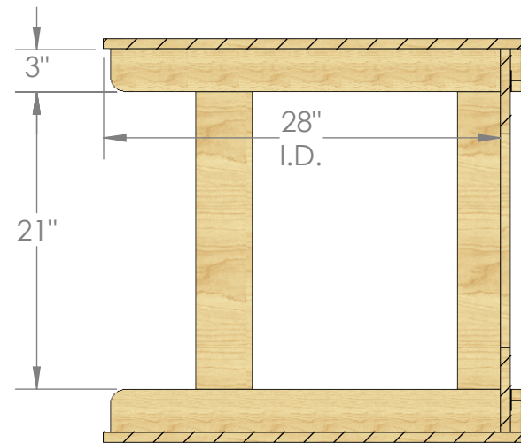
SECTION B-B SCALE 1 : 12
